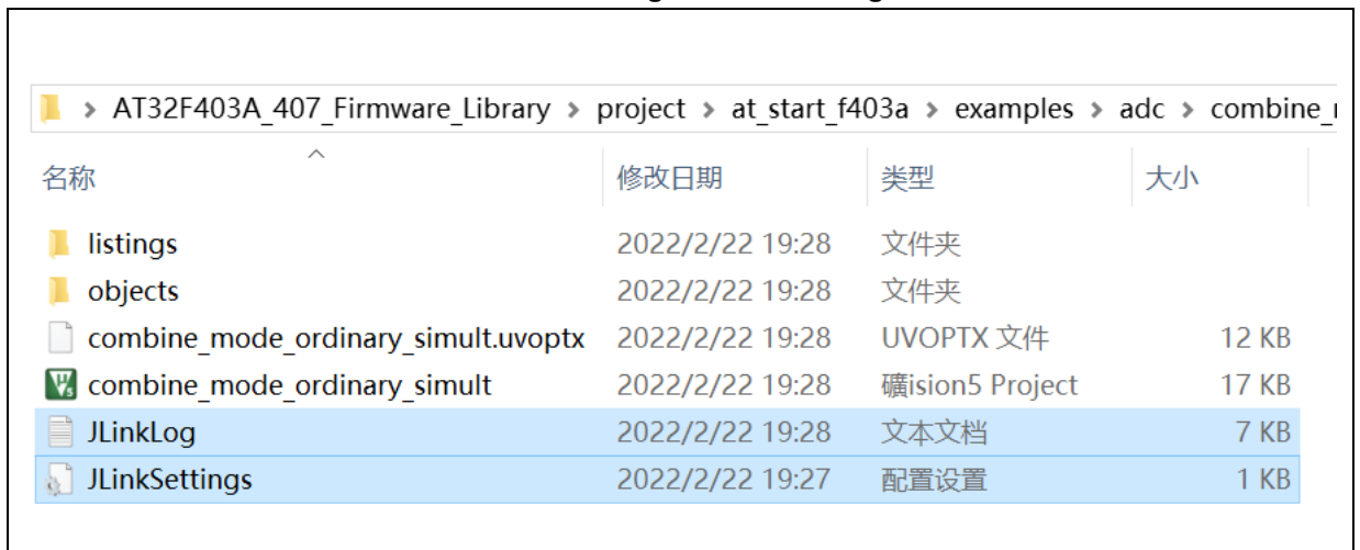
图 36. JLinkLog 和 JLinkSettings
