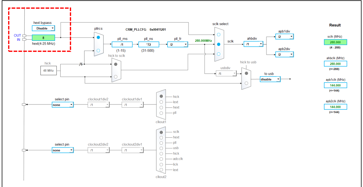
图 38. AT32_New_Clock_Configuration 界面
